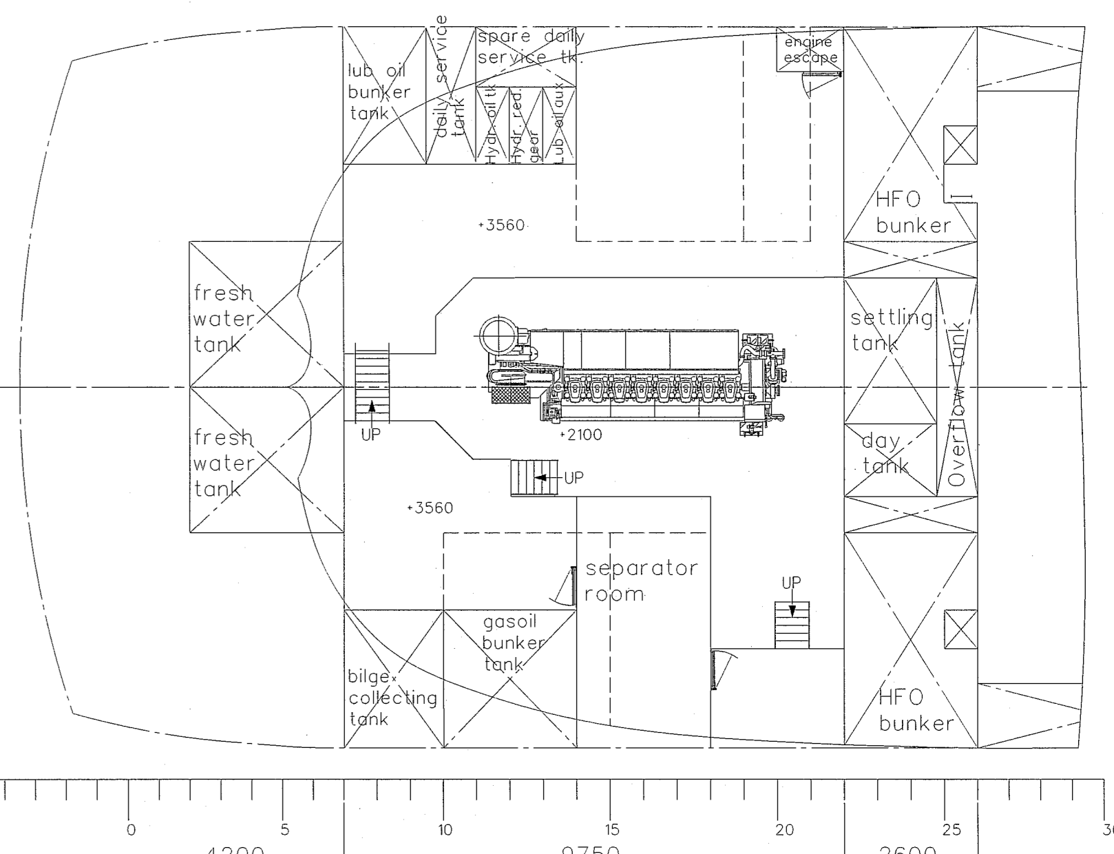
Tween Deck
