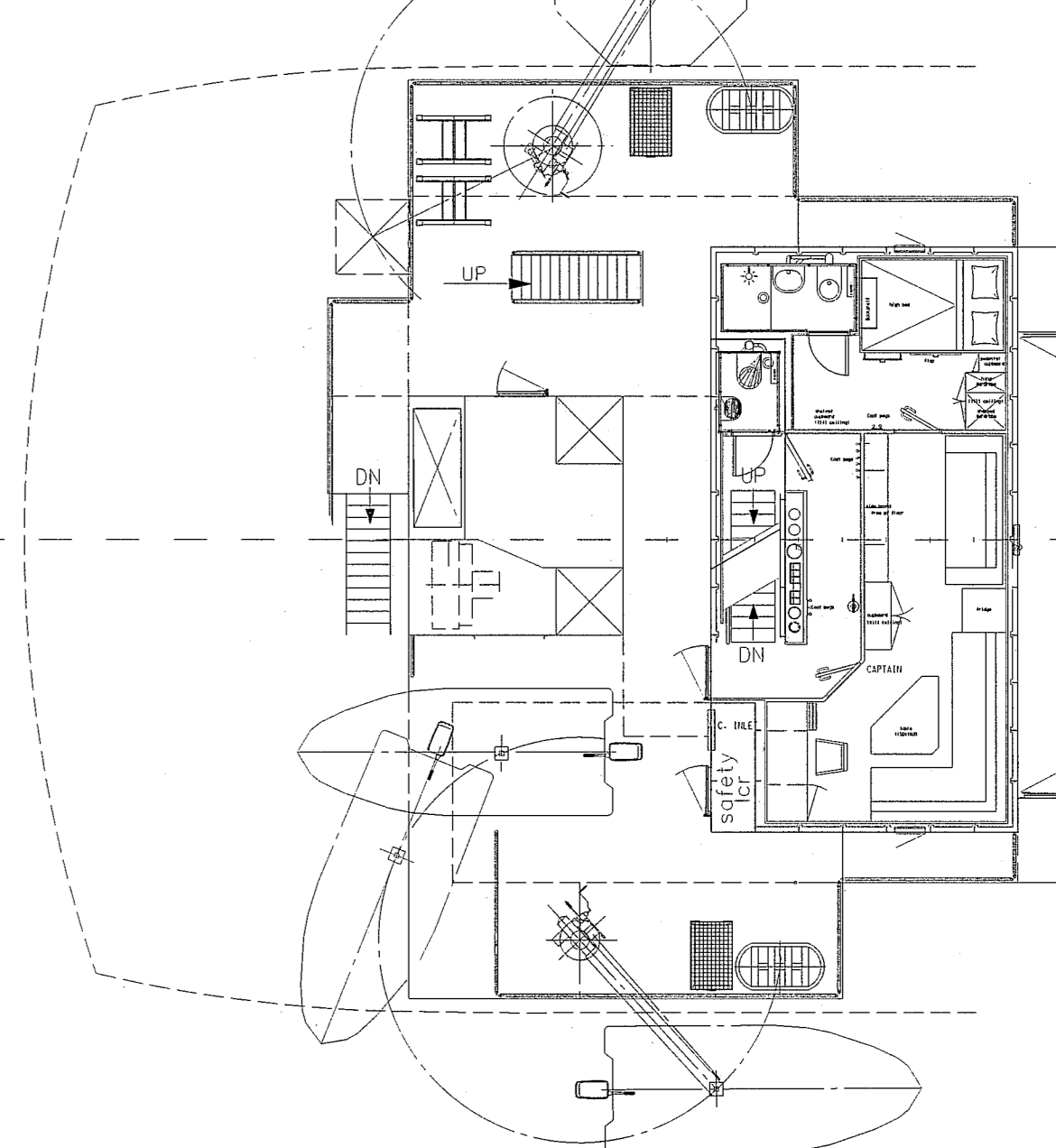
Tween Deck
